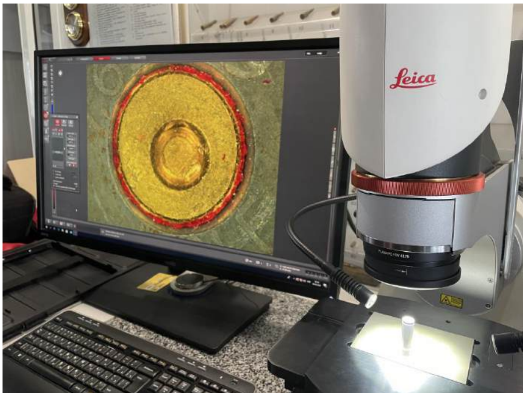
Гільза із слідами частин зброї на предметному столі мікроскопа Leica M80.
