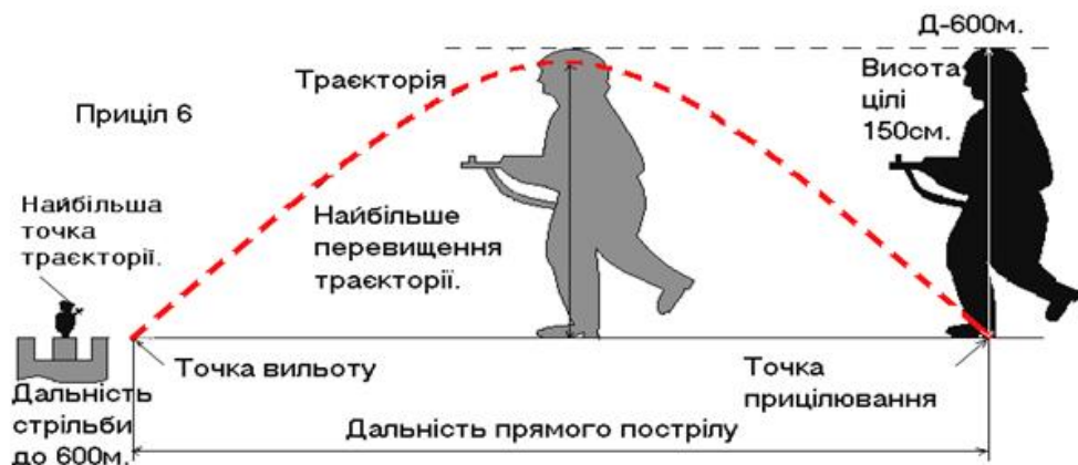
Рисунок 4.32 – Прямий постріл.
